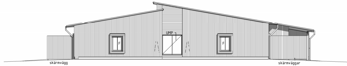
FASAD MOT ÖSTER
