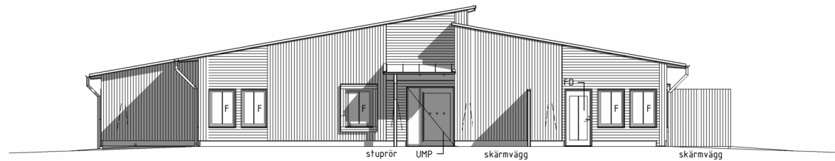
FASAD MOT VÄSTER
